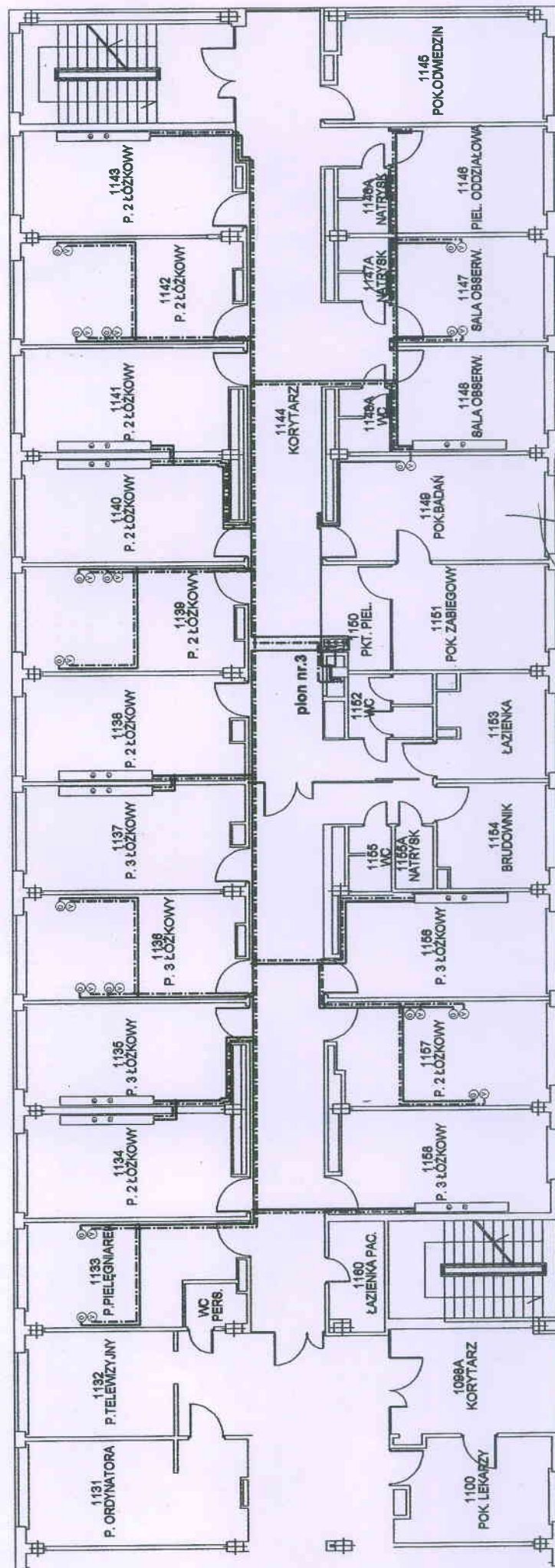
plan nr.3 możliwość oddzielenia pom. 1130 do 1146 do 1148 jednocześnie możliwość oddzielenia pom. 1130 do 1146 do 1148 jednocześnie możliwość oddzielenia pom. 1148 niezależnie
